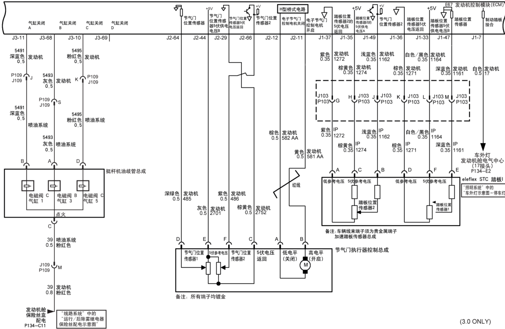
发动机控制系统示意图—3.0升V6
